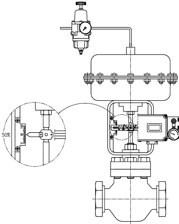
SP740 (스탠다드 레버 타입)
