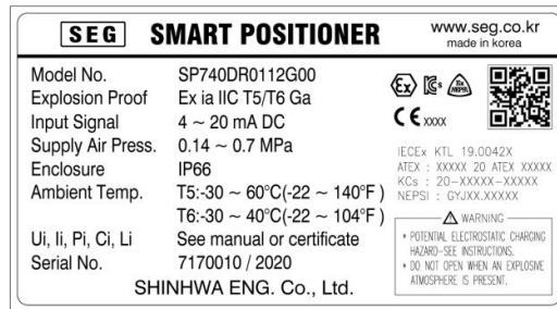
그림 2: SP740 본질안전 방폭 명판
