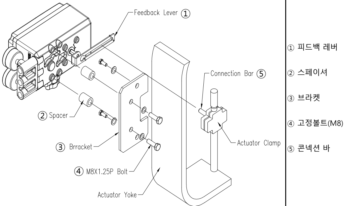
SP740 스탠다드 레버 타입
