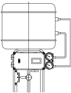
복동식 리니어 액추에이터
