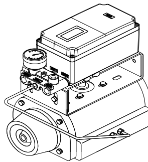
단동식 로터리 액추에이터
