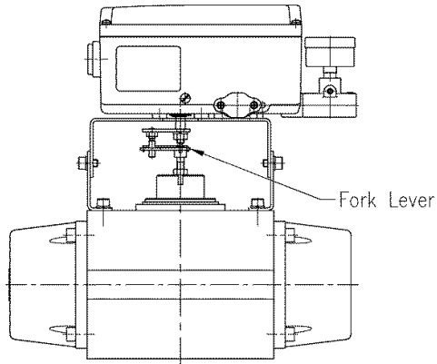
SP740 포크레버 타입
