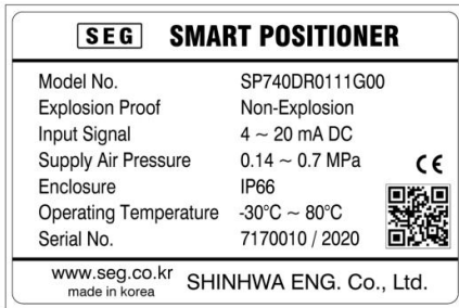
그림 1: SP740 비방폭 명판
