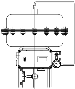
단동식 리니어 액추에이터
