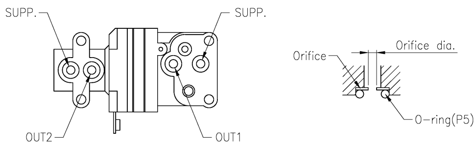
그림 6-4 : 오리피스 설치방법
