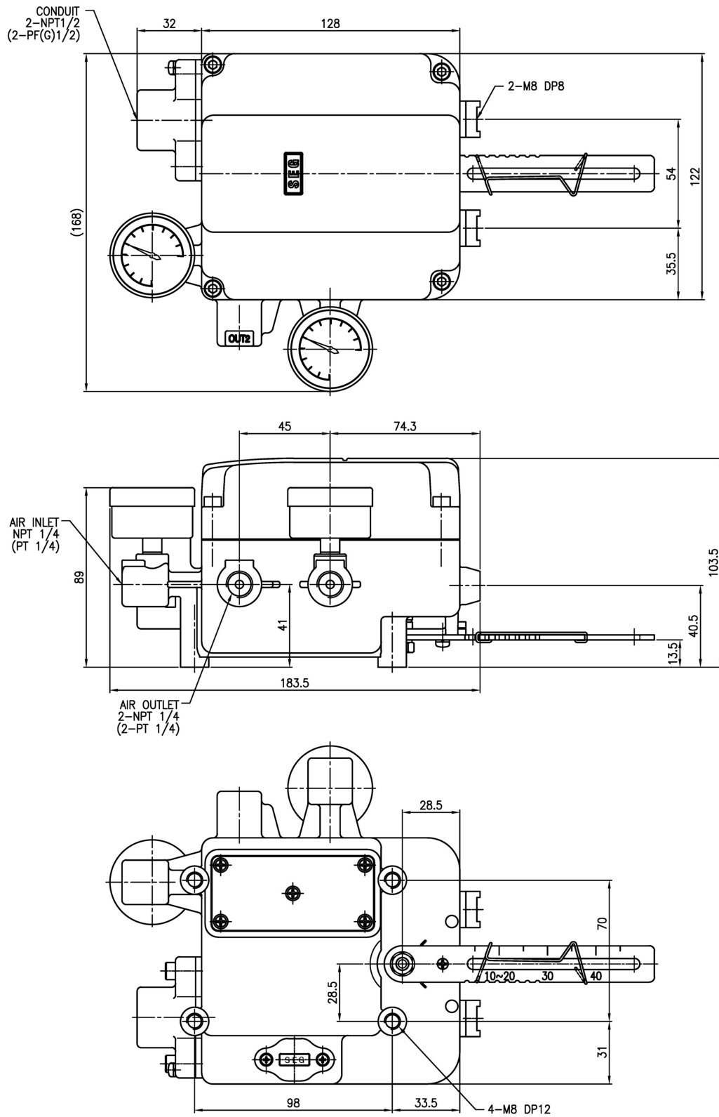
그림 2-9 : SP520 LINEAR TYPE (비방폭)
