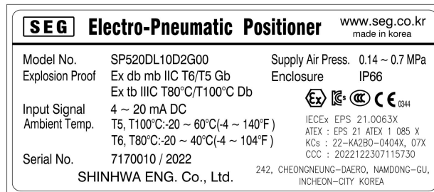
그림 2-4 : SP520 방폭표시 명판 (Ex db mb)
