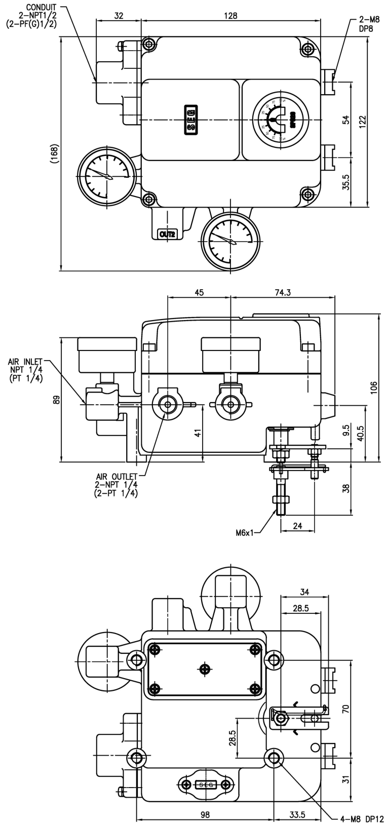
그림 2-11 : SP520 ROTARY TYPE (비방폭)
