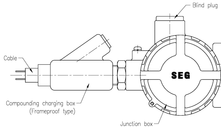
그림 5-2 : 컴파운드 충전방식 내압방폭형 전선관
