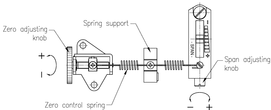
그림 6-1 : SPAN 조절 및 ZERO 구조
