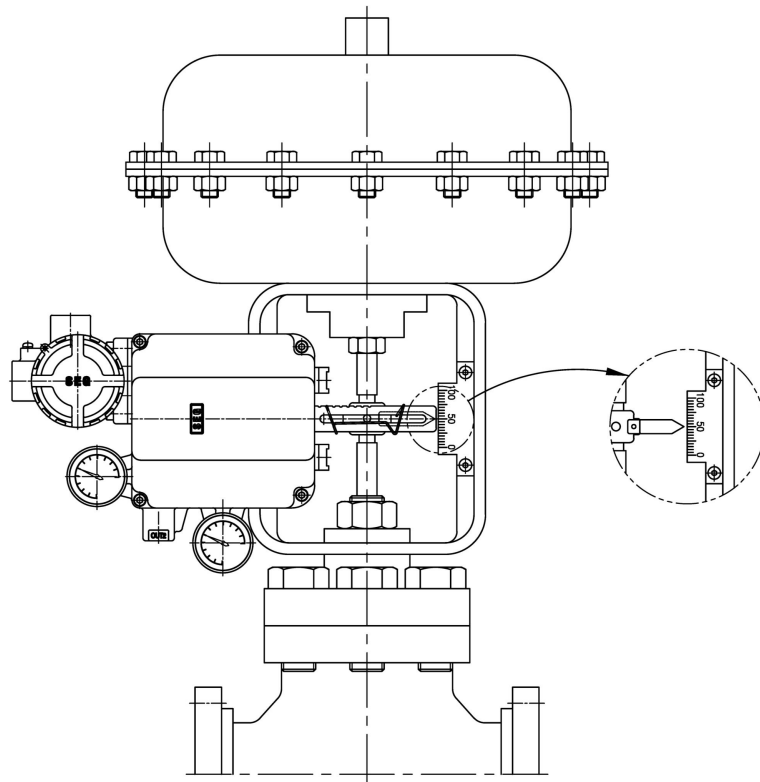
그림 3-3 : SP520 액추에이터에 포지셔너 설치하기
