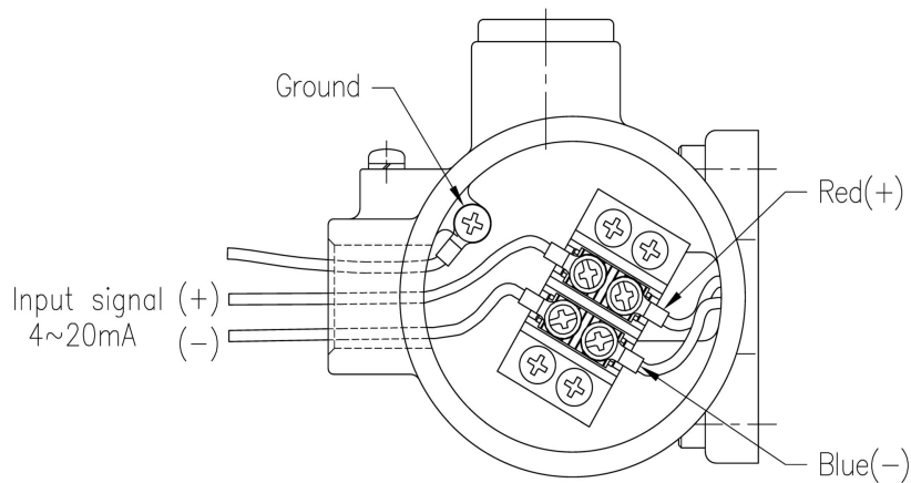
그림 5-6 : 내압방폭형, 본질안전형(무옵션) 전원단자의 연결
