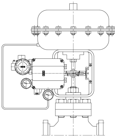
그림 4-1 : 단동식 리니어 액추에이터
