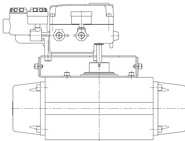
그림 3-10 : 나무어 타입 설치
