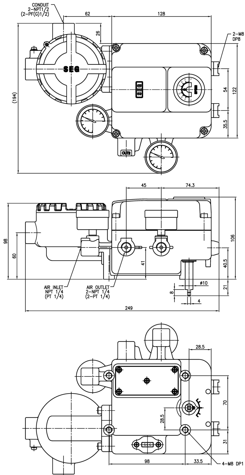
그림 2-13 : SP520 ROTARY TYPE (NAMUR, FEEDBACK OPTION)
