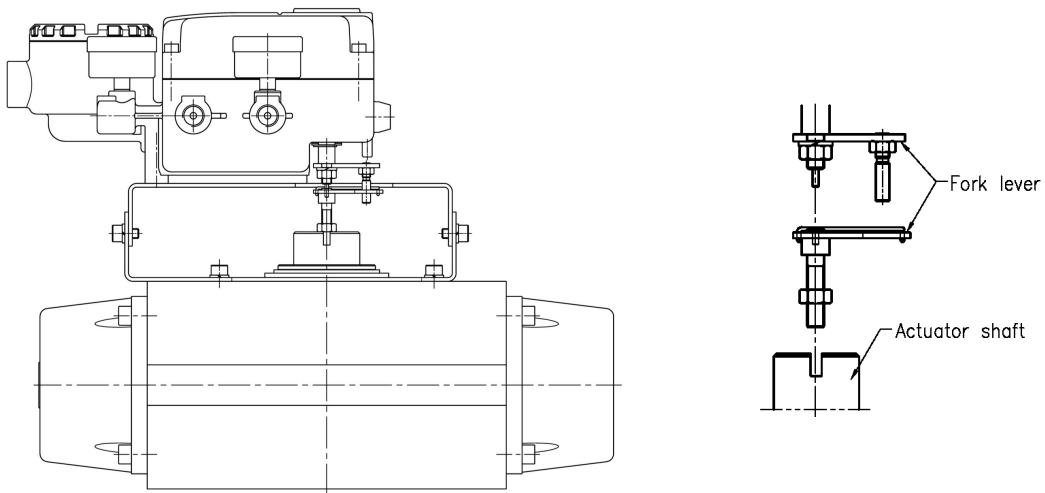
그림 3-9 : 포크레버 타입 설치
