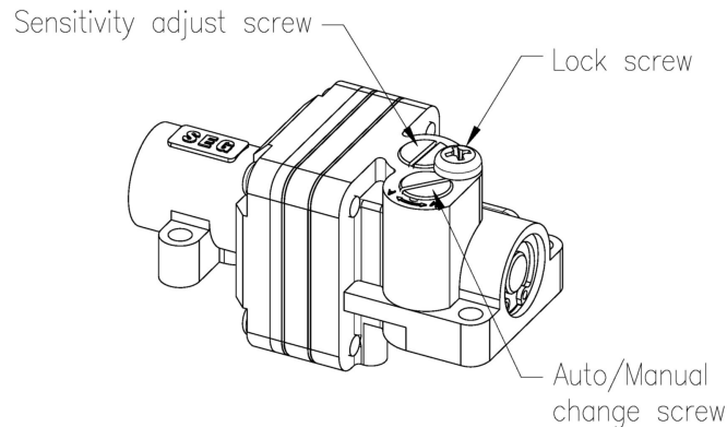
그림 6-3 : 오토/매뉴얼 전환 나사
