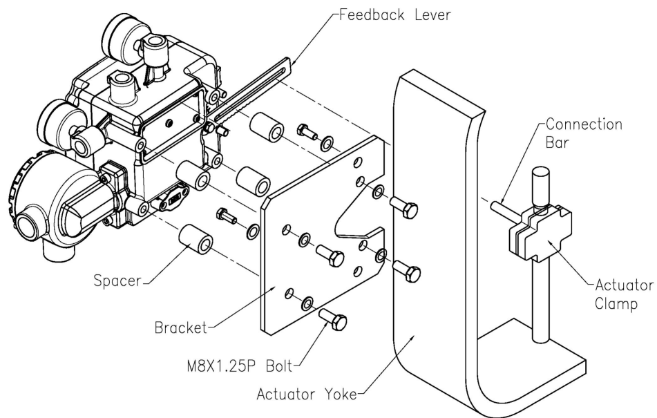
그림 3-2 : SP520 액츄에이터에 포지셔너 설치하기
