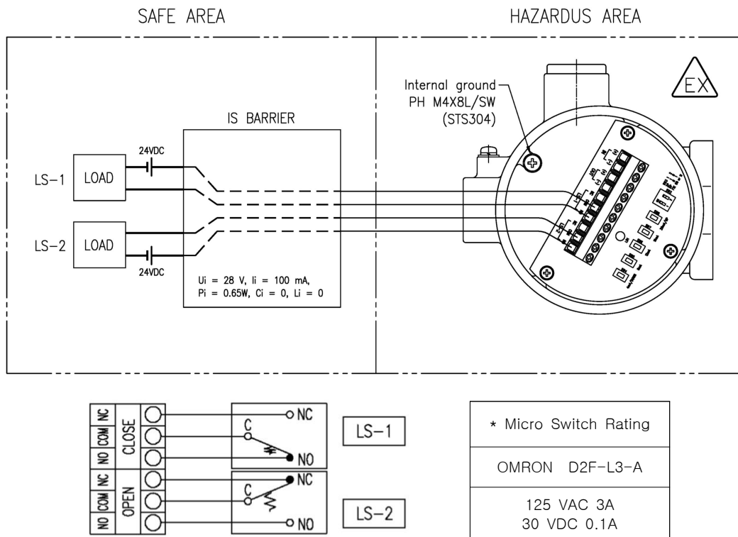
그림 5-9 : 본질안전형(FEEDBACK+LIMIT SWITCH 옵션) 전원단자의 연결
