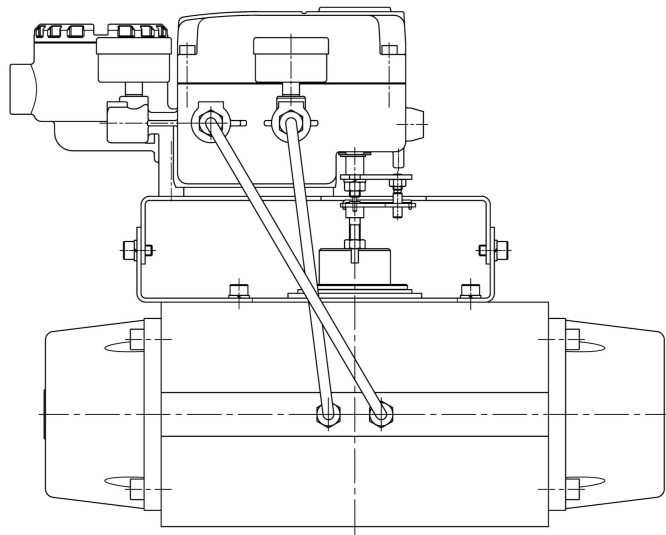
그림 4-4 : 복동식 로터리 액츄에이터
