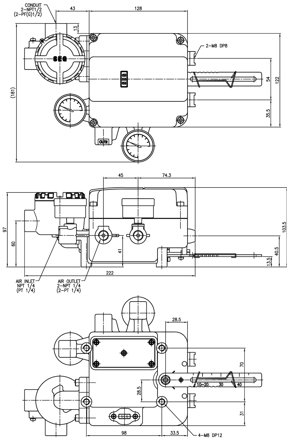
그림 2-10 : SP520 LINEAR TYPE (방폭)
