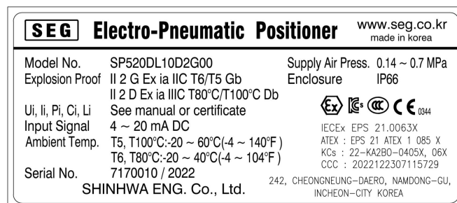
그림 2-2 : SP520 방폭표시 명판 (Ex i)
