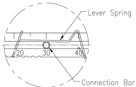
그림 3-4 : 레버와 스프링 사이에 연결봉 삽입방법 (스트로크 30mm)
