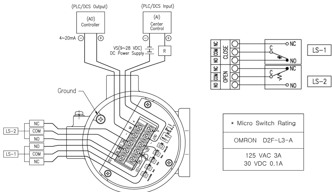
그림 5-5 : 비방폭형(FEEDBACK+LIMIT SWITCH 옵션) 전원단자의 연결
