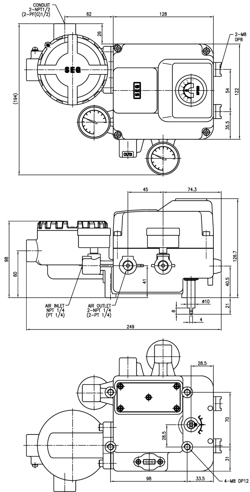
그림 2-14 : SP520 ROTARY TYPE (LIMIT SWITCH OPTION)
