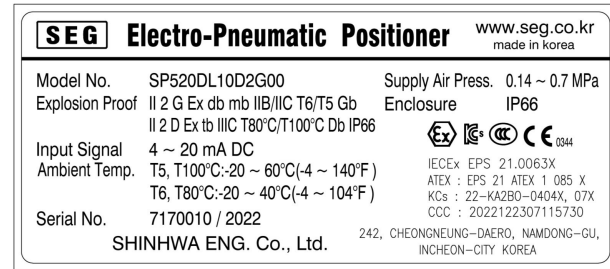
그림 2-3 : SP520 방폭표시 명판 (Ex db mb)
