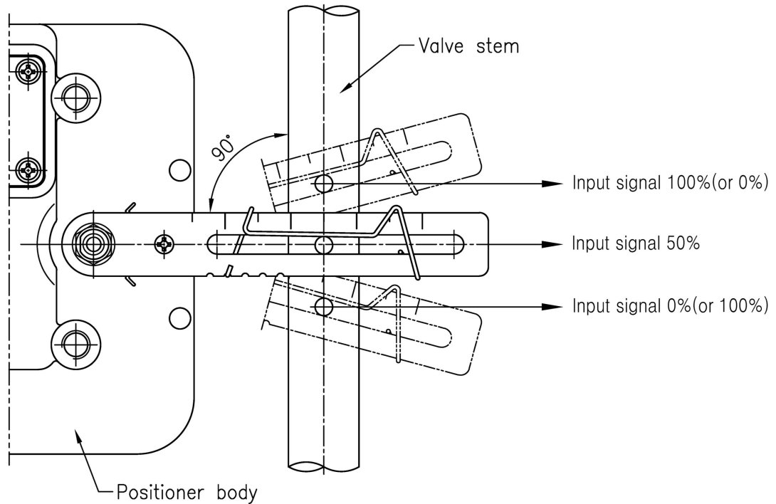
그림 3-5 : 밸브 위치가 50%일 때 수평으로 설치된 레버
