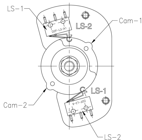
그림 6-2 : 기계식 리미트 스위치 동작 위치 조절
