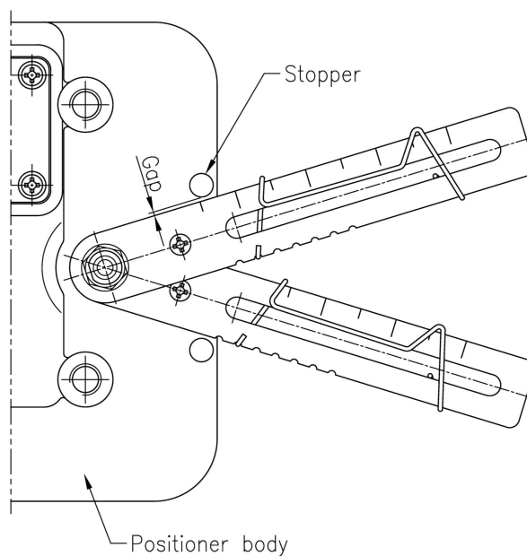
그림 3-8 : SP520 레버와 스토퍼의 틈새
