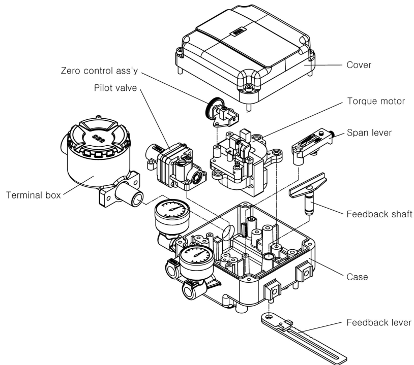
그림 2-7 : LINEAR TYPE 분해도
