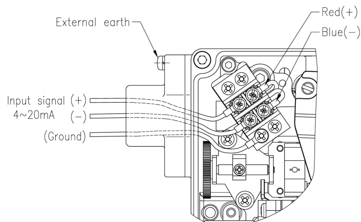
그림 5-3 : 비방폭형(무오픈) 전원단자의 연결
