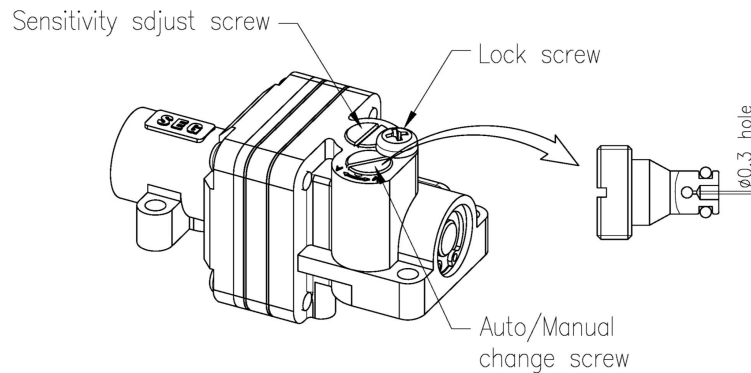
그림 6-5 : 오토/매뉴얼 전환 나사의 세척
