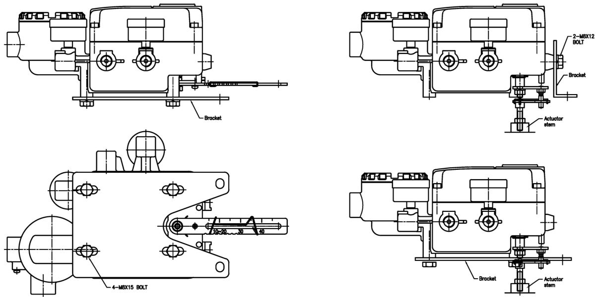
그림 3-7 : SP520 브라켓 설치 방법
