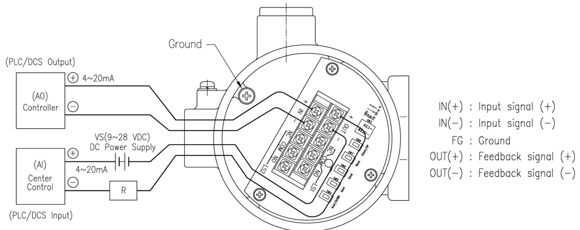
그림 5-4 : 비방폭형(FEEDBACK 옵션) 전원단자의 연결
