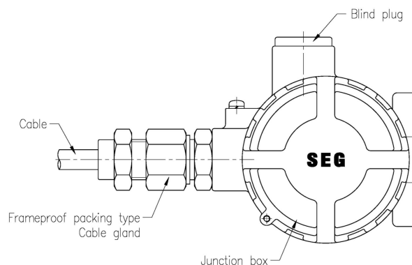
그림 5-1 : 내압 방폭형 전선관
