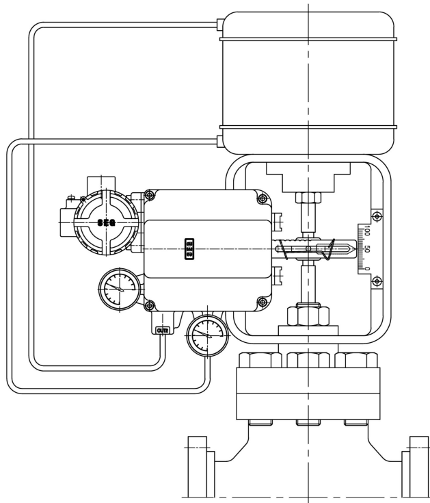
그림 4-3 : 복동식 리니어 액츄에이터
