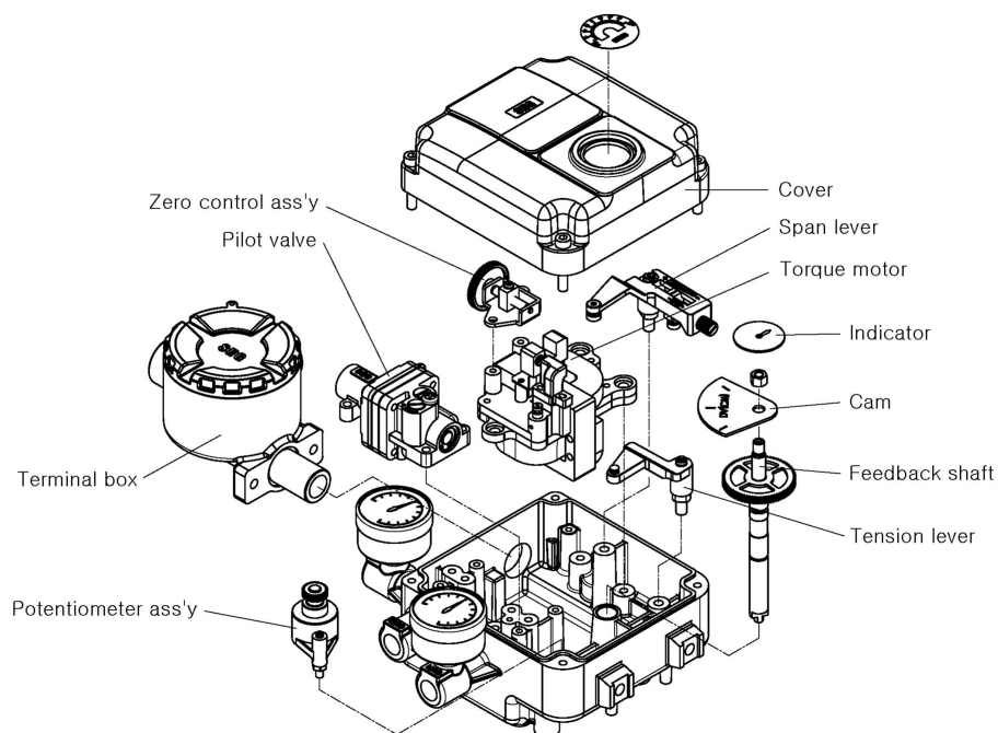
그림 2-8 : ROTARY TYPE 분해도
