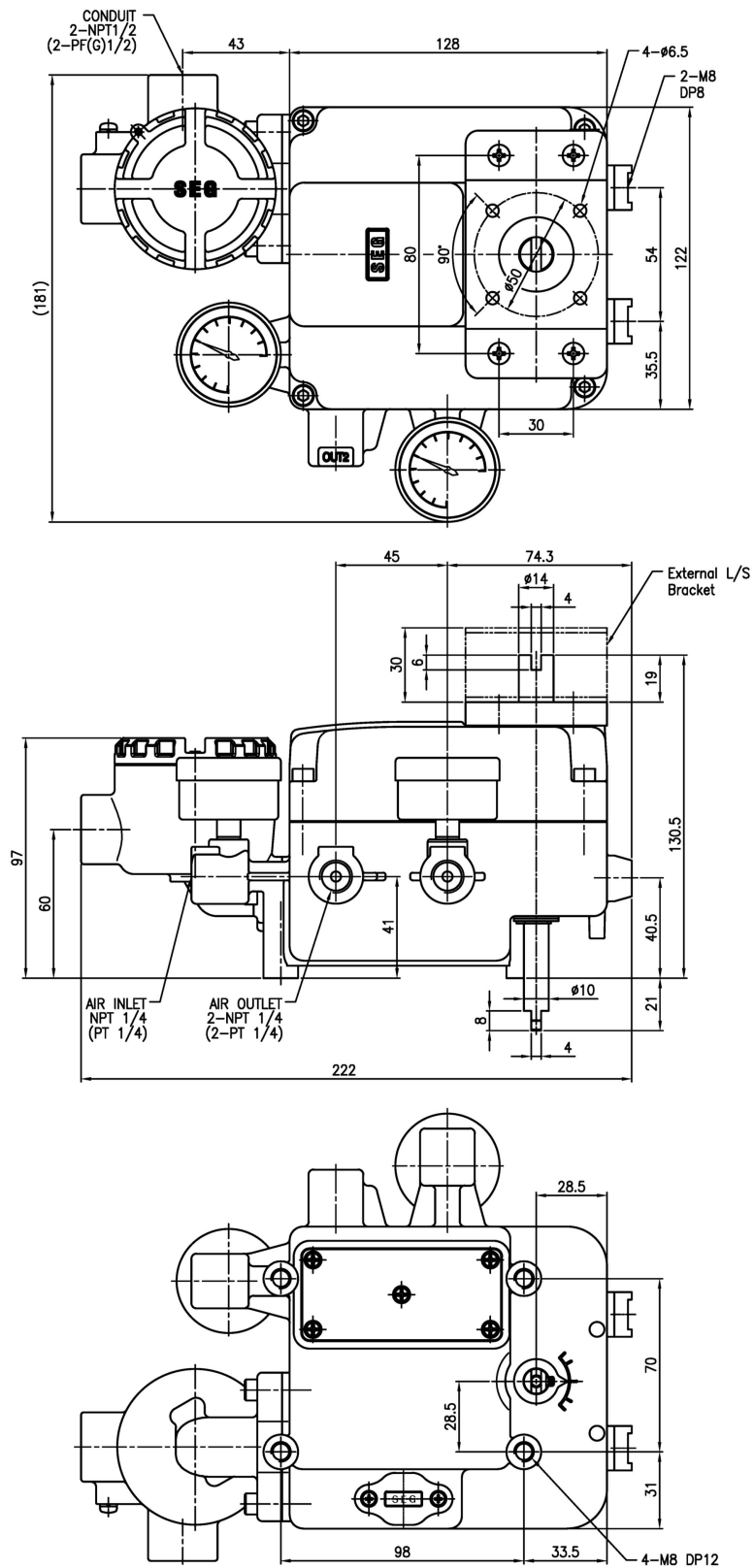
그림 2-15 : SP520 ROTARY TYPE (외장 L/S + 외장 FEEDBACK OPTION)
