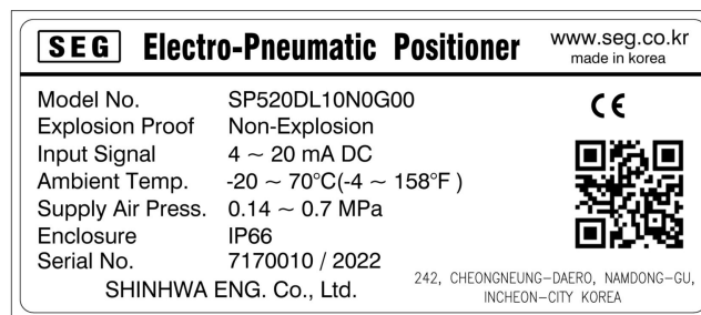
그림 2-1 : SP520 스티커 명판
