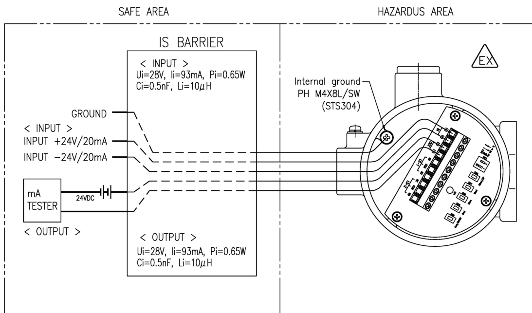
그림 5-7 : 본질안전형(FEEDBACK 옵션) 전원단자의 연결
