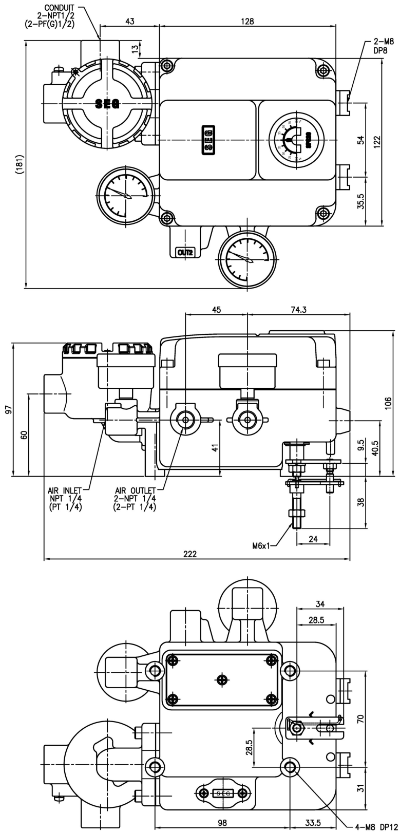
그림 2-12 : SP520 ROTARY TYPE (FORK LEVER)
