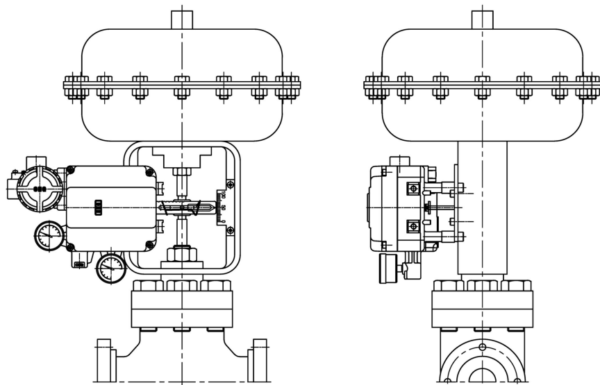
그림 3-1 : SP520 설치예
